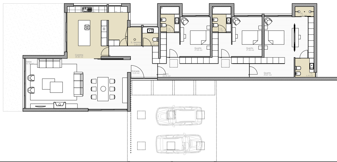
PLANTA PISO 0
