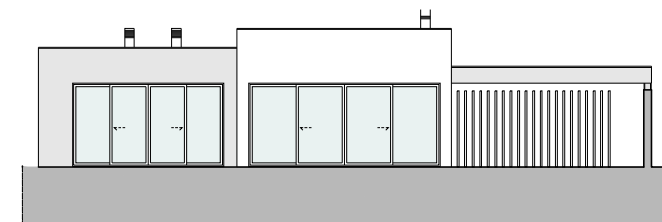
ALÇADO LATERAL 1
