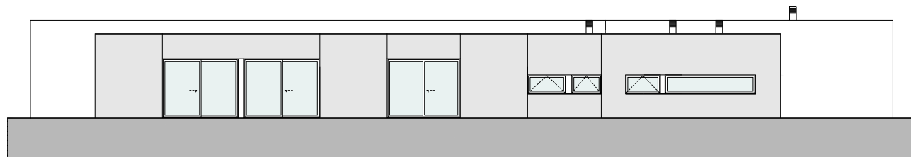
ALÇADO TARDOZ
